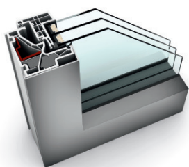
KF 500 PLASTHLINÍKOVÉ OKNO
