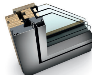
HF 410 DŘEVOHLINÍKOVÉ OKNO
