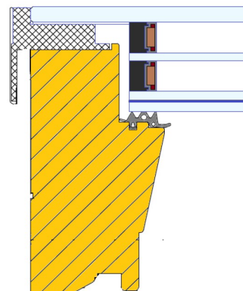
Obr. 1: Řez okna FNF P6
