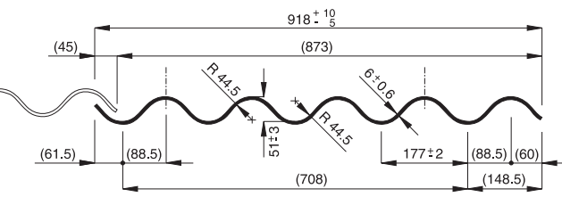
Vlnitá krytina A5
